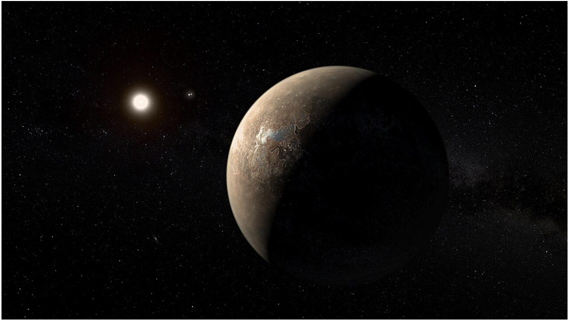
Próxima b
